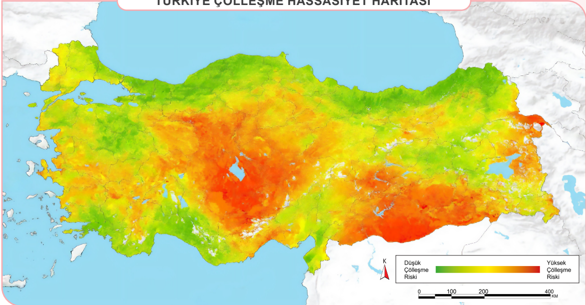
Harita 2.6 Türkiye Çölleşme Hassasiyet Haritası
